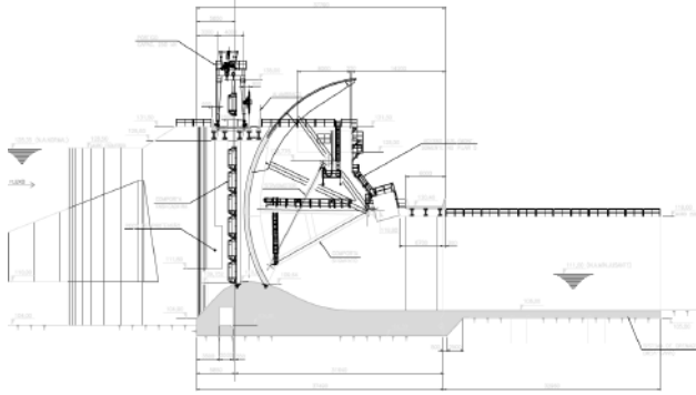
Пример необходимого чертежа - боковой разрез
