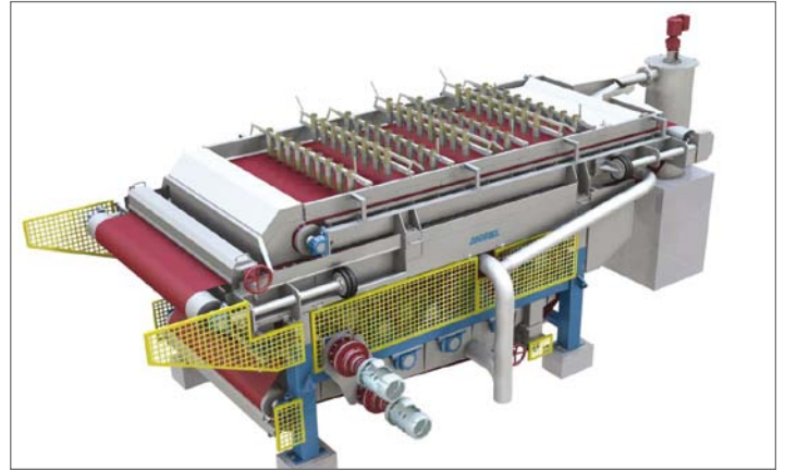
▲ CPF犀牛浓缩机(带有预脱水重力区)用于对生物物质含量达到100%的污泥进行脱水
