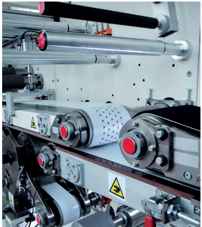
D-TECH 口罩生产线的内视图
