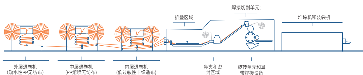
安德里茨 D-TECH 口罩生产线布局
