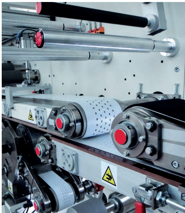
D-TECH フェイスマスクラインの内部
