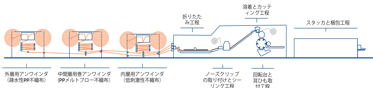
ANDRITZ D-TECH フェイスマスク製造設備レイアウト
