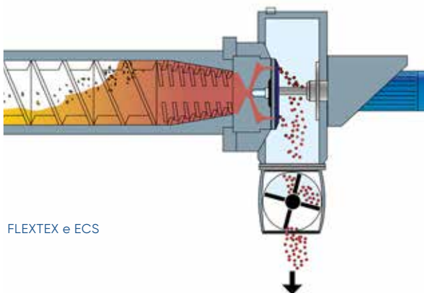
Extrusora com ECS instalado
